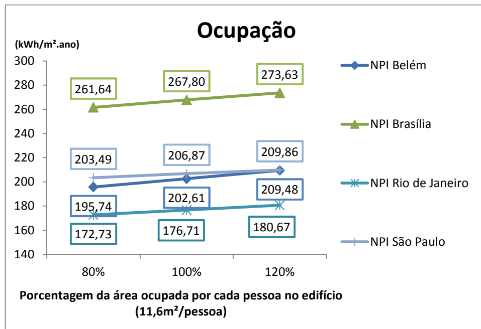
Figura 5.7 – NPI em função do parâmetro de ocupação
