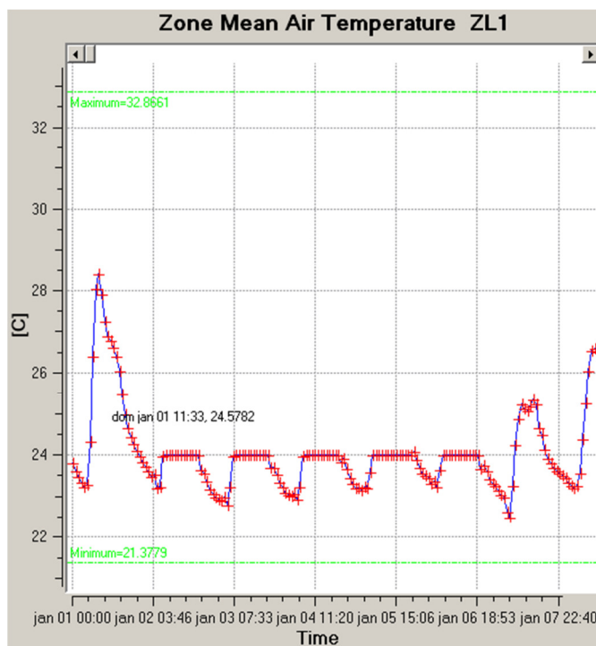
Figura 3.3 – Temperatura na zona térmica de face leste do andar térreo no edifício de referência. Simulação para o clima de São Paulo.
