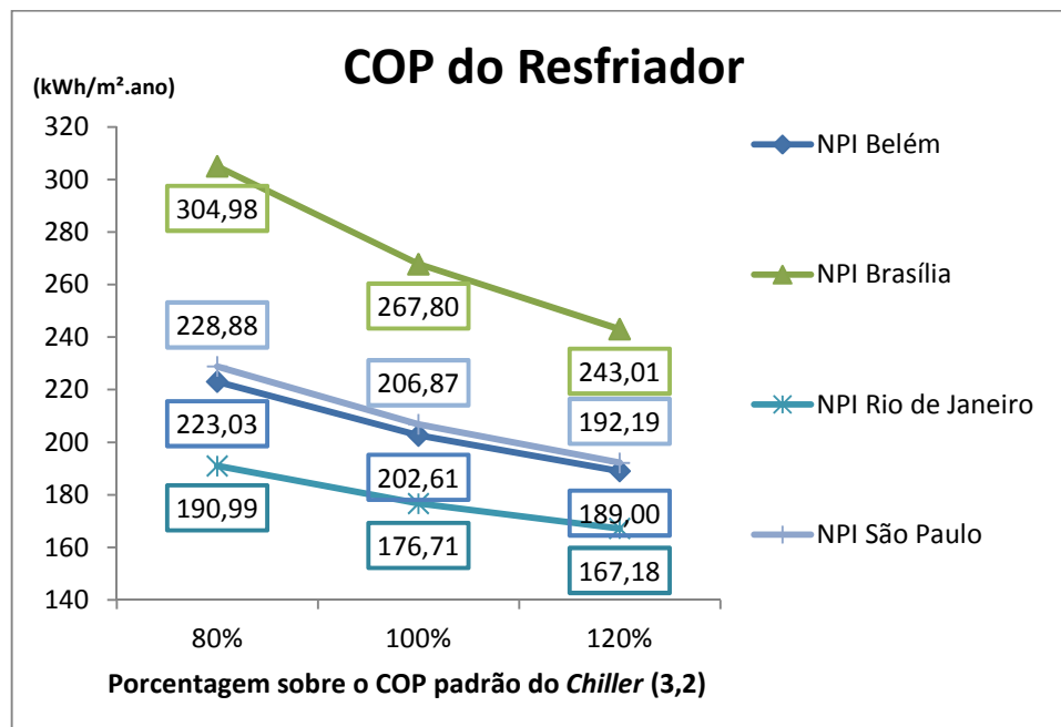
Figura 5.3 –NPI em função do COP do Resfriador
