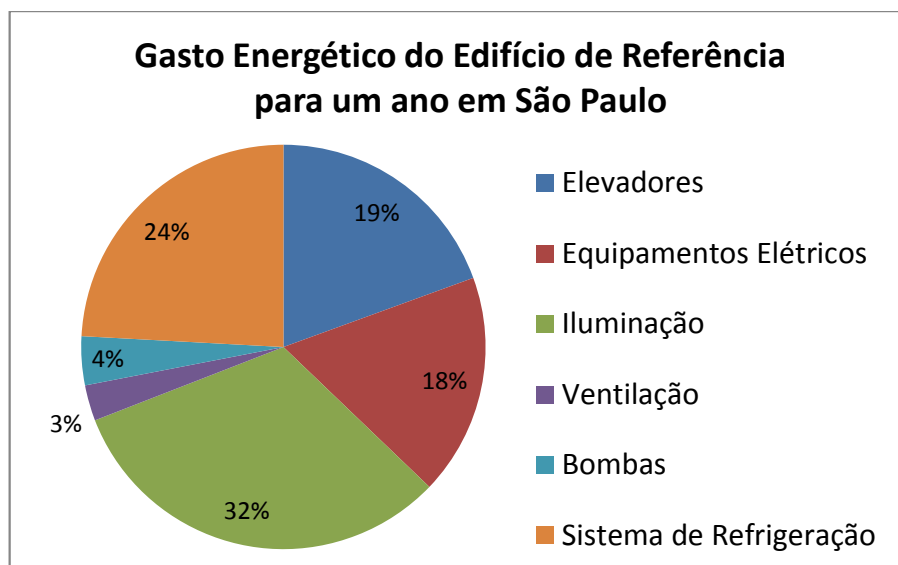
Figura 4.1 – Consumo elétrico do edifício simulado por tipo de equipamento, em um ano, para o arquivo de clima de São Paulo, Congonhas
