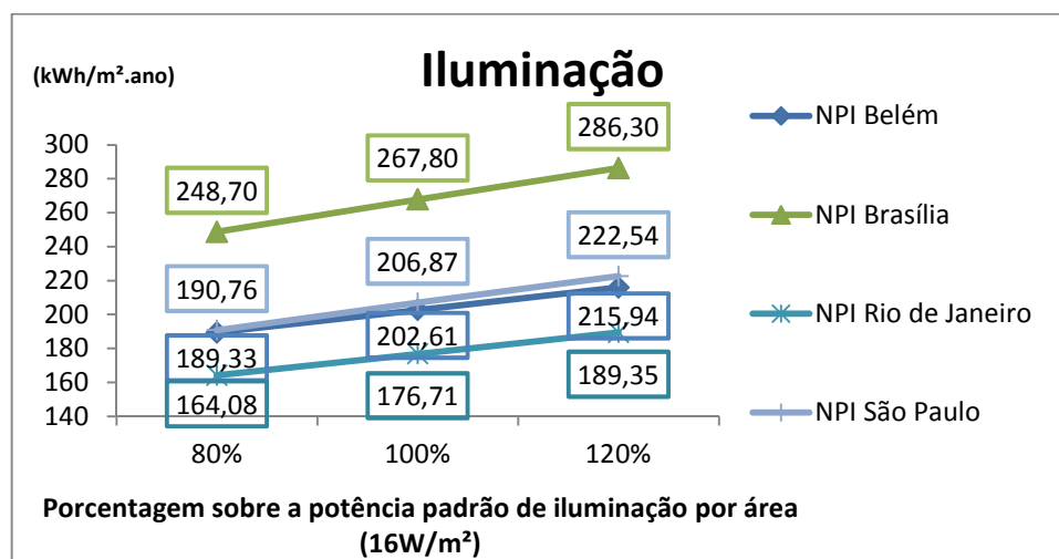
Figura 5.1 – NPI em função do parâmetro de luminosidade
