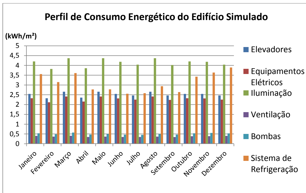
Figura 4.3 – Perfil de Consumo Elétrico do Edifício Simulado, para o arquivo de clima de São Paulo, Congonhas (U.S. Department of Energy, 2009)
