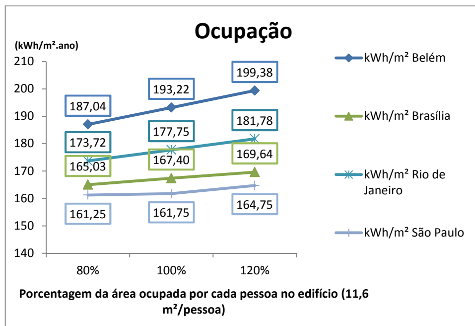
Figura 5.8 – Consumo elétrico sobre área em função do parâmetro de ocupação
