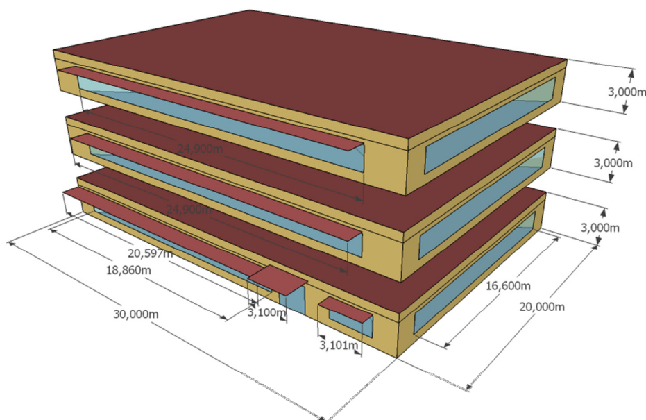
Figura 3.1 – Modelo Tridimensional dos três andares típicos utilizados no modelo computacional.
