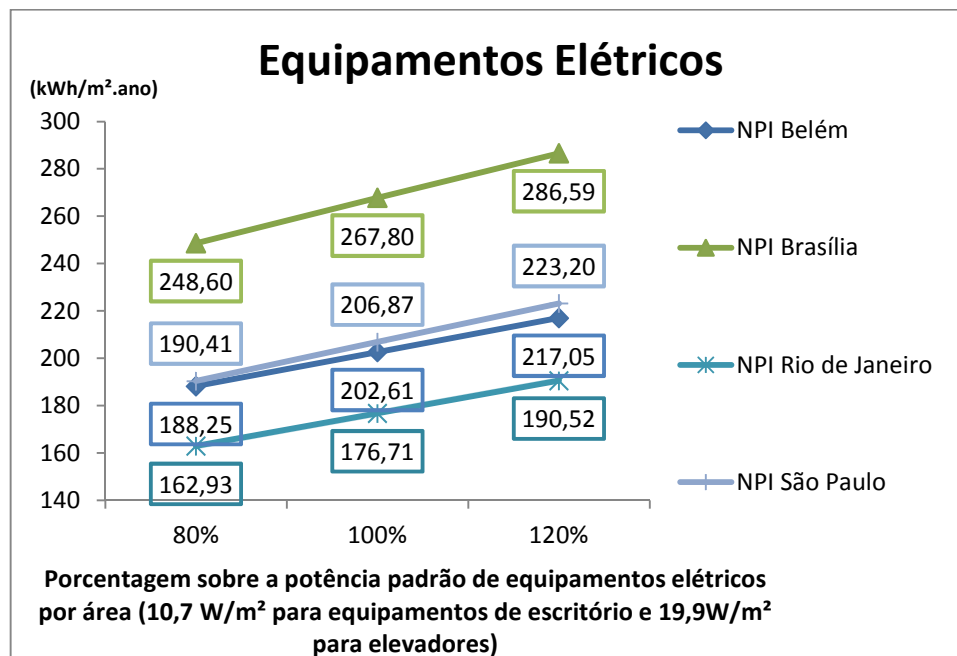
Figura 5.5 –NPI em função da variação da potência utilizada por equipamentos elétricos
