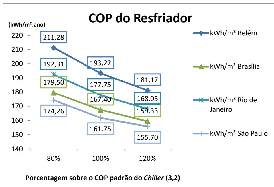
Figura 5.4 – Consumo elétrico sobre a área em função do COP do Resfriador
