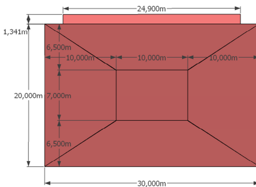
Figura 3.2 – Zonas térmicas e brises de um pavimento do edifício
